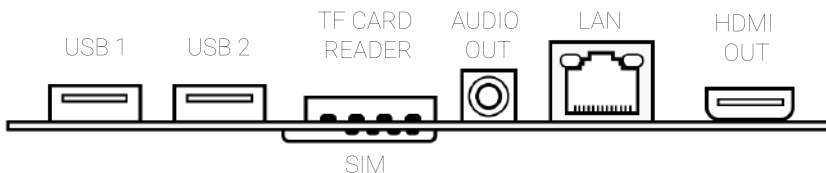
Рис. Вид интерфейсной части мониторов оборудованных платформой RK 3288 (2Gb/8Gb) (выпускается серийно)
